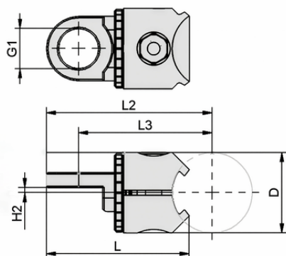
Dati di costruzione SAUG-ANB G3/8-IG 52.9 PXT
