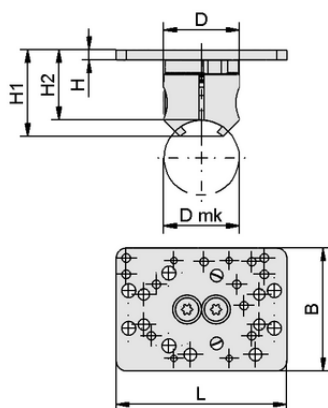
Datos de diseño HTR-D30-I AR PXT
