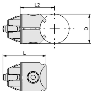
デザインデータ VBR-PR D30-I D30-I
