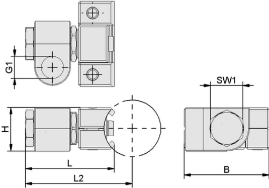
Tasarım verileri SAUG-ANB PXT D30-I ROT IV
