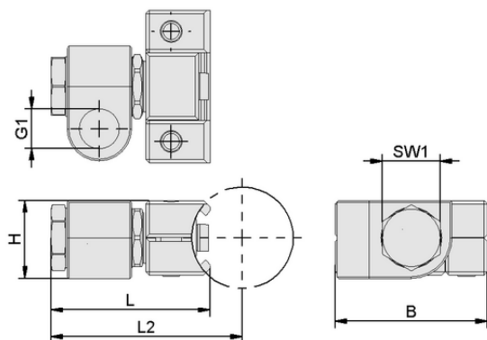
Конструктивные данные SAUG-ANB PXT D30-I ROT IV
