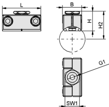
Конструктивные данные SAUG-ANB G1/4-IG 42 PXT
