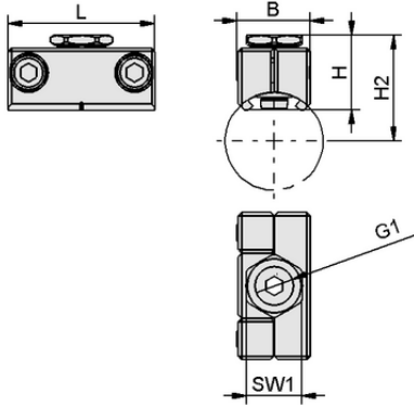
Tasarım verileri SAUG-ANB G1/4-IG 42
