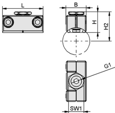
Datos de diseño SAUG-ANB G1/4-IG 42
