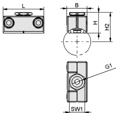
デザインデータ SAUG-ANB G1/4-IG 42
