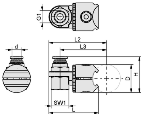
Конструктивные данные SAUG-ANB PXT D30-I ROT
