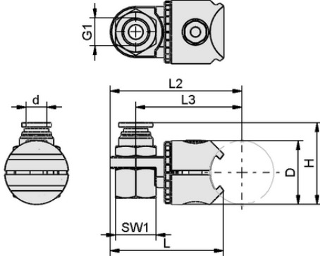
Tasarım verileri SAUG-ANB PXT D30-I ROT
