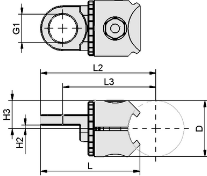
Tasarım verileri HTR-D30-I M16x1-IG FSTE PXT
