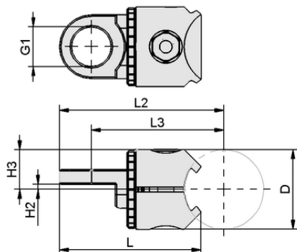
Datos de diseño HTR-D30-I M16x1-IG FSTE PXT
