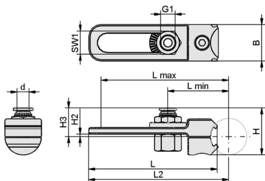
デザインデータ SAUG-ANB PXT D30-I SH
