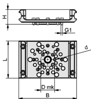
Datos de diseño SET PXT 64 2LT FANUC
