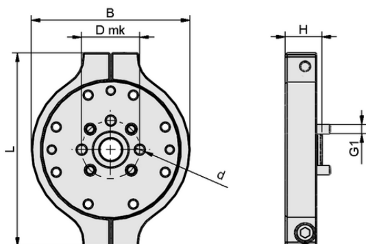
Datos de diseño SET PXT 63 9409-1 1LT YASKAWA
