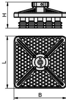
Datos de diseño RFBP 50 50 BA SPB2
