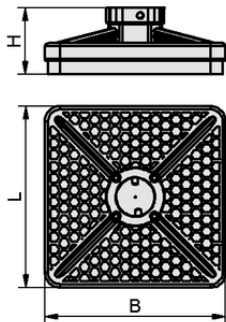
Données de construction RFBP 100 58 BA O10
