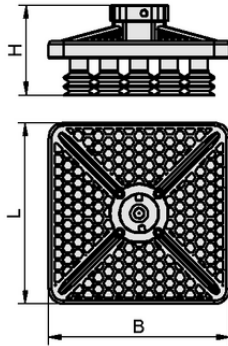
Tasarım verileri RFBP 120 120 BA SPB2
