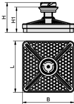
Données de construction RFBP 120 120 O10
