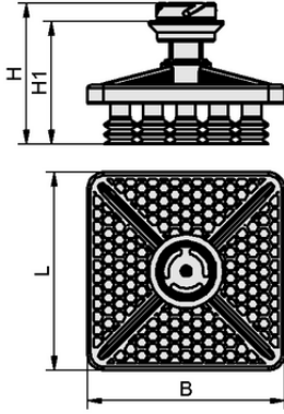
Tasarım verileri RFBP 120 120 SPB2
