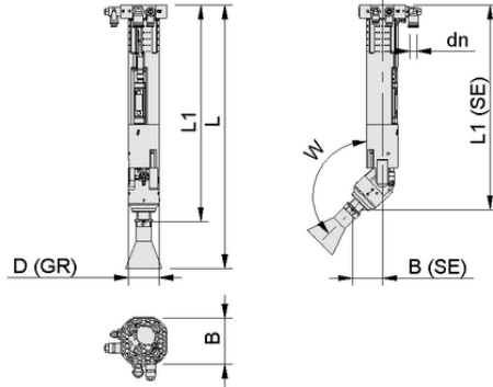
Tasarım verileri SBPG-SET M PSE QS 50
