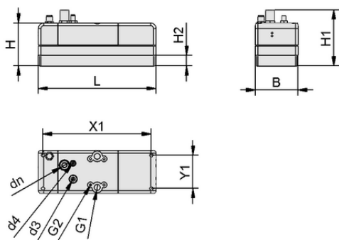
Dati di costruzione FQE Xc 220x80 SW130 O20
