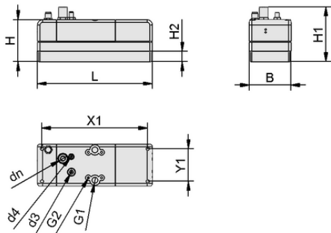
Design data FQE Xc 220x80 SW130 O20
