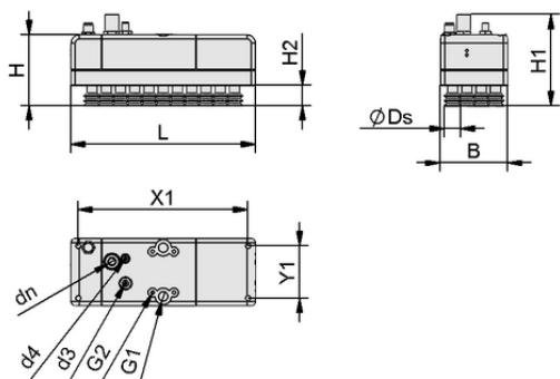
Datos de diseño FQE Xc 220x80 SW130 SPB2
