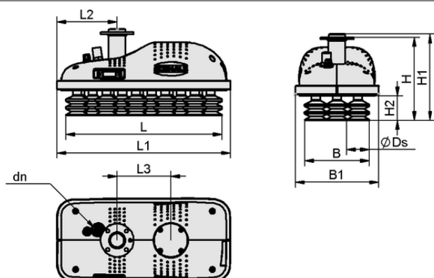
Données de construction ROB-SET FXCB DOOSAN SPB2
