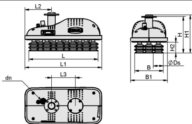
Datos de diseño ROB-SET FXCB YASKAWA SPB2
