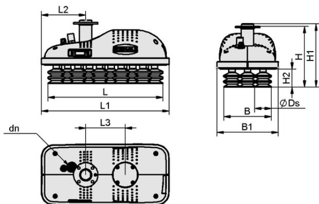
Données de construction ROB-SET FXCB YASKAWA SPB2
