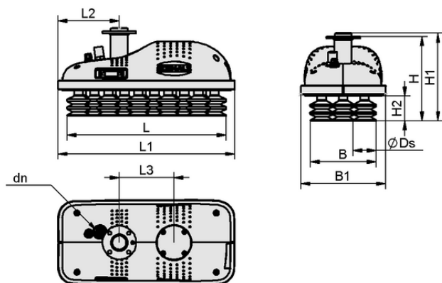
デザインデータ ROB-SET FXCB FANUC SPB2
