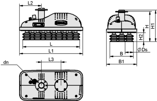
Tasarım verileri ROB-SET FXCB KUKA SPB2
