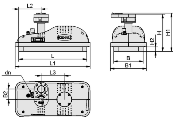
Datos de diseño ROB-SET FXCB OMRON O20
