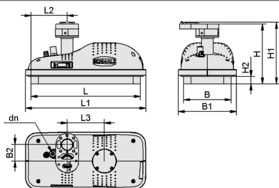
Dati di costruzione ROB-SET FXCB TECHMAN O20
