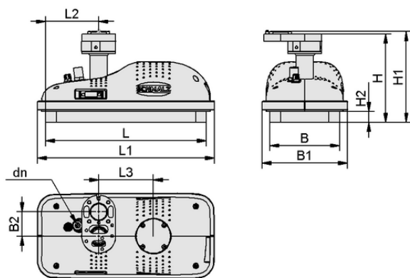
Données de construction ROB-SET FXCB TECHMAN O20
