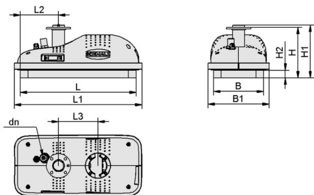
Données de construction ROB-SET FXCB FANUC O20
