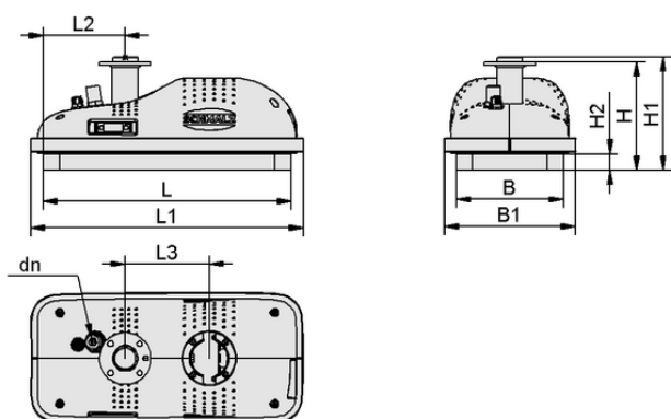
Dati di costruzione ROB-SET FXCB KUKA O20
