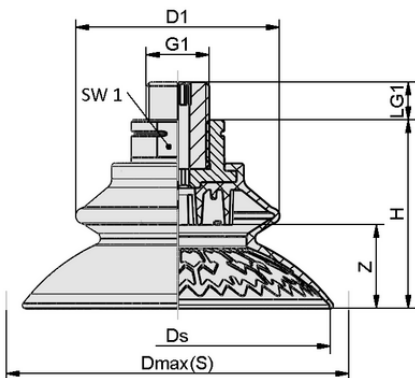
Datos de diseño SAXB 120 ED-85 M10-AG
