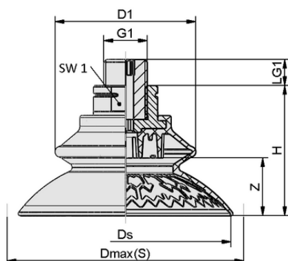
デザインデータ SAXB 120 ED-85 G3/8-AG
