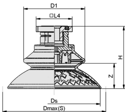
Datos de diseño SAXB 100 ED-85 RA
