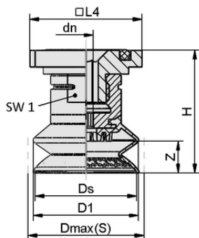
Dati di costruzione SAXB 40 ED-85 RA
