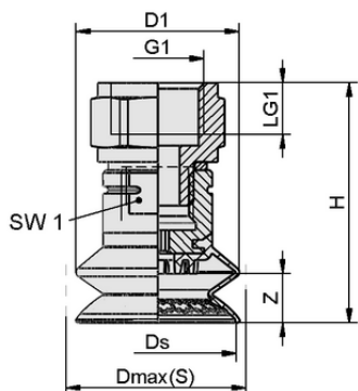
Datos de diseño SAXB 40 ED-85 NPT3/8-IG
