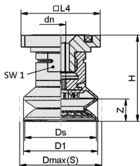
Dati di costruzione SAXB 30 ED-85 RA
