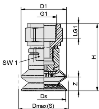
Dati di costruzione SAXB 20 ED-85 G3/8-IG
