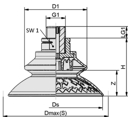
デザインデータ SAXB 60 ED-85 M16-AG
