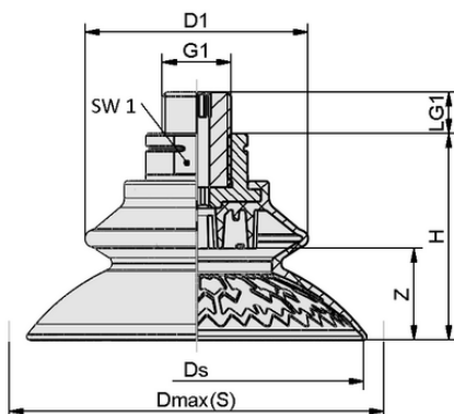
Données de construction SAXB 60 ED-85 M16-AG
