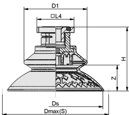
Datos de diseño SAXB 80 ED-85 RA
