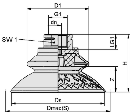
Datos de diseño SAXB 80 ED-85 G3/8-IG
