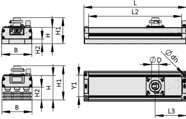
Tasarım verileri FA-Mi SVK 442 3R54 SPB2-40P
