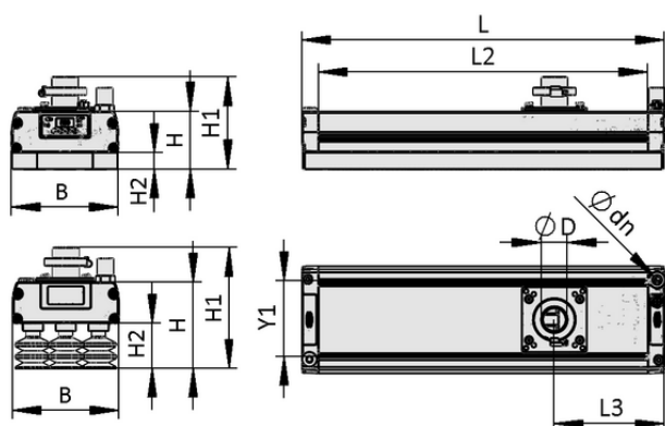
デザインデータ FA-Mc SVK 442 3R54 SPB2-40P
