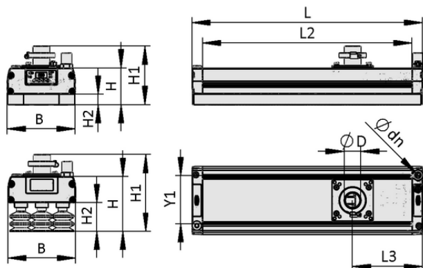
Dati di costruzione FA-Mc SVK 442 3R54 SPB2-40P
