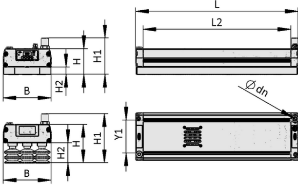
Tasarım verileri FA-Xb SVK 442 3R54 SPB2-40P
